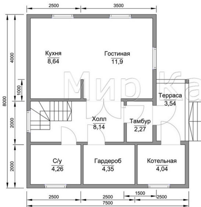
План 1-ого этажа
